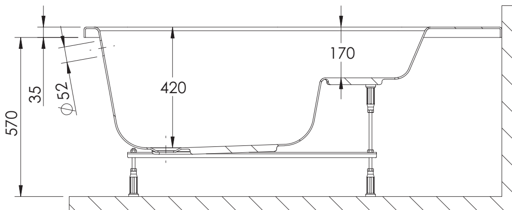
ŘEZ A-A
